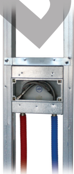
Exemplo aplicação em pladur | Application exemple in plaster board walls | Ejemplo de aplicación en pared de cártón-yeso | Exemple d'application en plaques de plâtre
